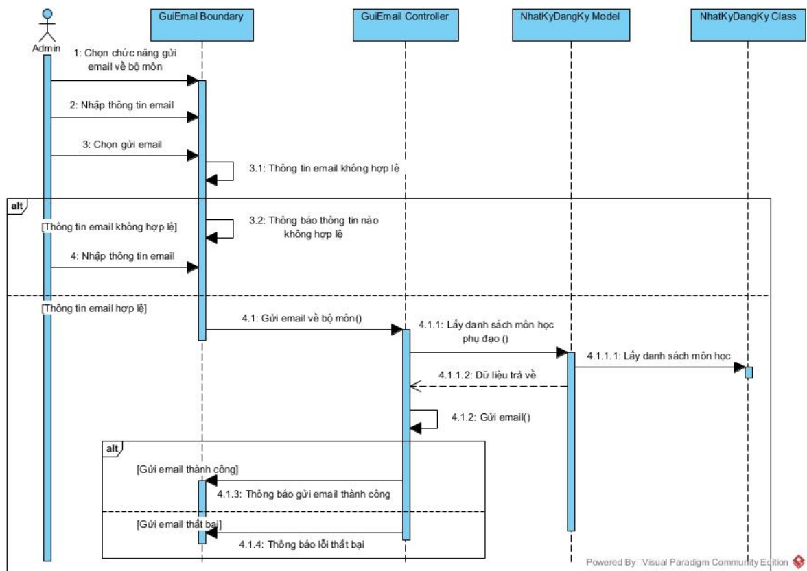
Hình 11: Biểu đồ tuần tự chức năng Gửi email về bộ môn
