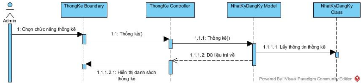
Hình 10: Biểu đồ tuần tự chức năng Thống kê đợt phụ đạo
